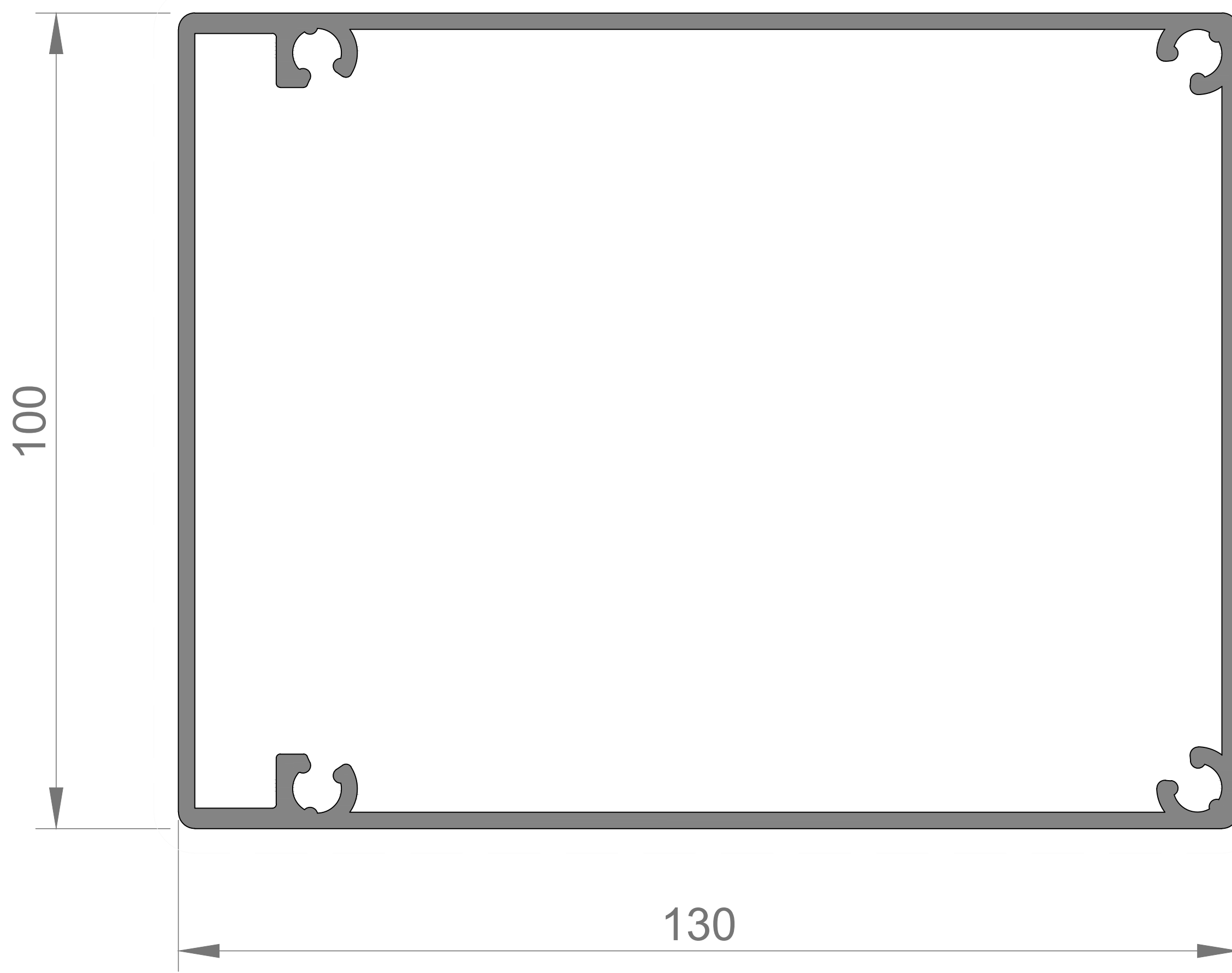
DİKME PROFİLİ 8471 2.767 kg/mt
