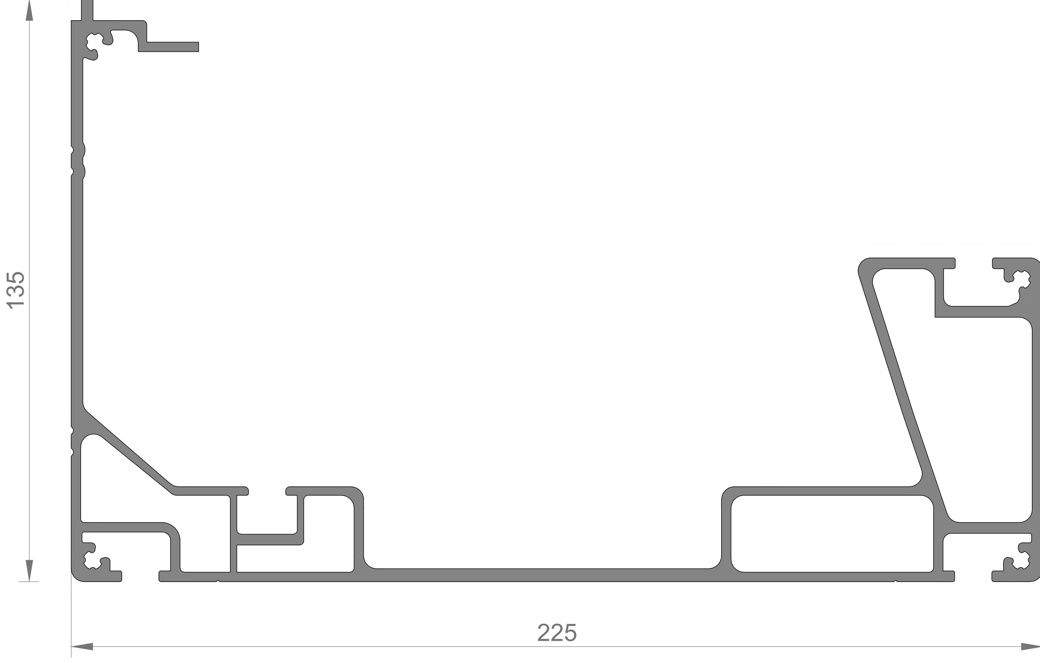
DERE PROFİLİ 3344 5.600 kg/mt
