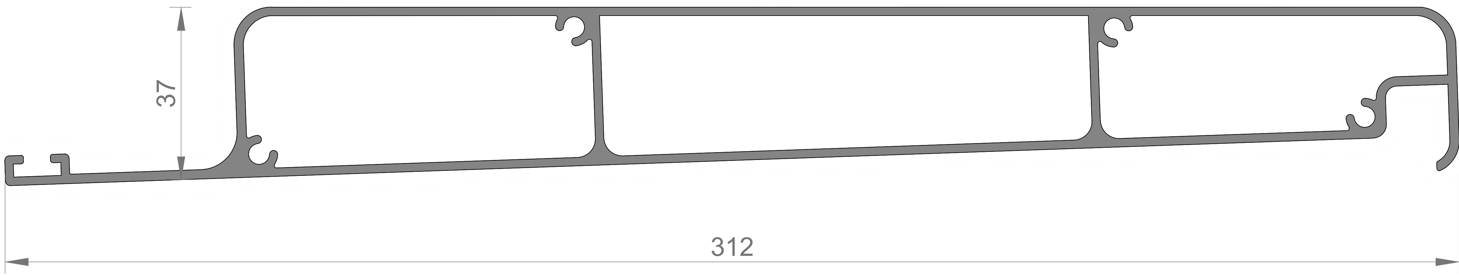
HAREKETLİ PANEL PROFİLİ 7383 3.833 kg/mt
