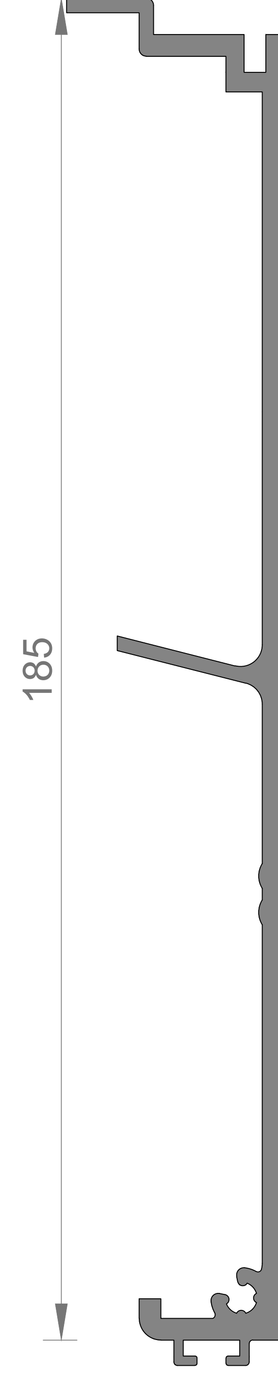
DERE KAPAK PROFİLİ 3345 1.950 kg/mt
