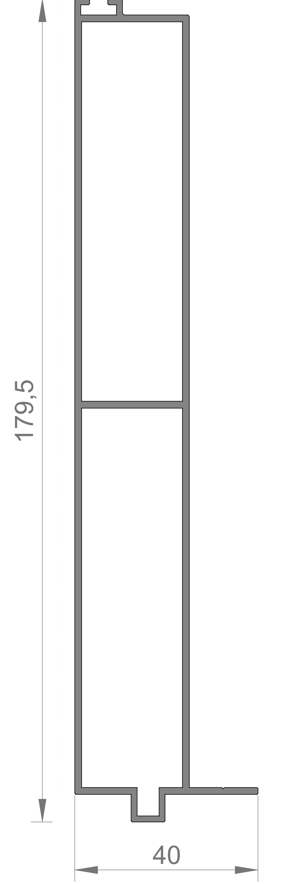
DERE İÇ KAPAMA PROFİLİ 8469 1.786 kg/mt
